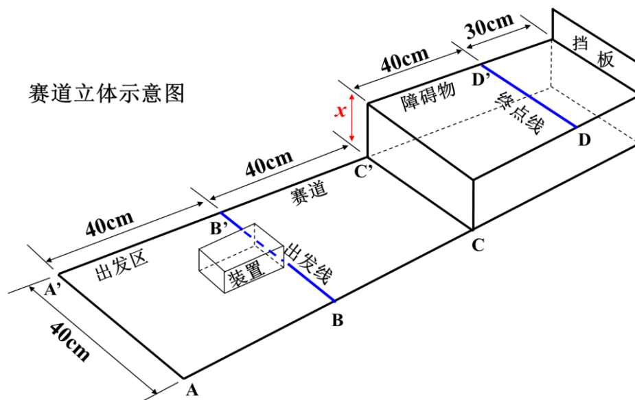
图 1 初赛赛道立体示意图
